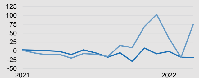
Spreads 1 (EUR/MWh)
